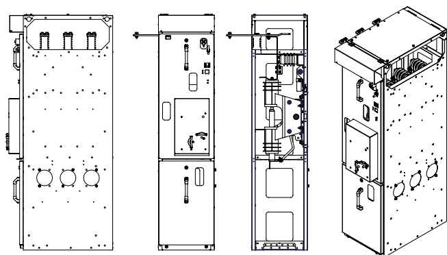
Рис. 6.4.2. Камера с ВН
