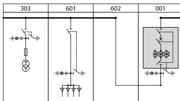
Рис. 8.1. Однолинейная схема кабельного ввода
