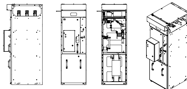
Рис. 6.3. Камера с ТСН
