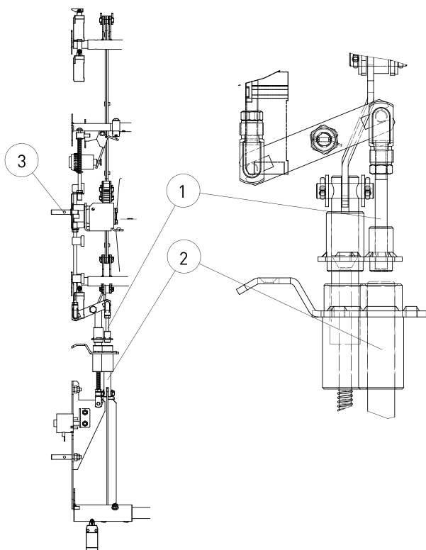
1 – Ось блокировки линейного и шинного разъединителя; 2 – Ось блокировки линейного заземлителя; 3 – Ручка доступа к окну управления линейным и шинным разъединителями.
