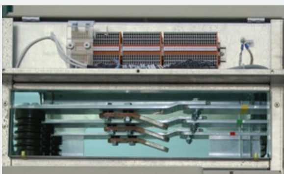
Рис. 5.13. Короб транзитных цепей
