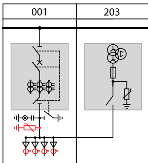
рис. 8.4. Индикация напряжения до ввода
