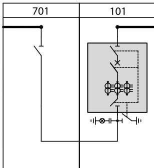
Рис. 8.3. Шинное секционирование
