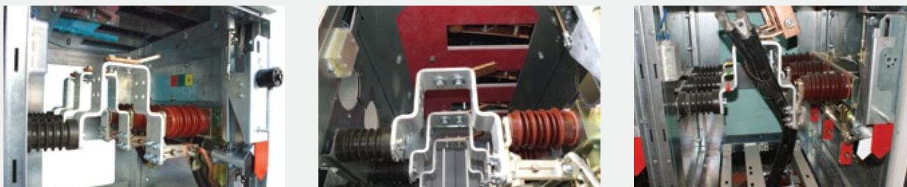
Рис. 5.8. Отсек присоединений
