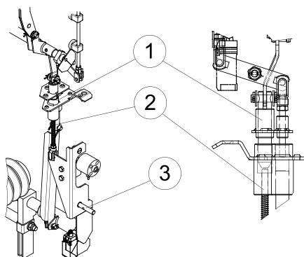
1 – Ось блокировки линейного и шинного разъединителя; 2 – Ось блокировки линейного заземлителя; 3 – Ручка доступа к окну управления линейным и шинным разъединителями.
