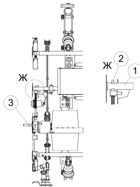
1 – Вал вакуумного выключателя (ВВ); 2 – Ось блокировки вала ВВ; 3 – Ручка доступа управлению разъединителями.
