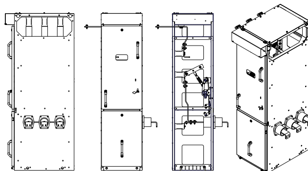
Рис. 6.5. Камера СР
